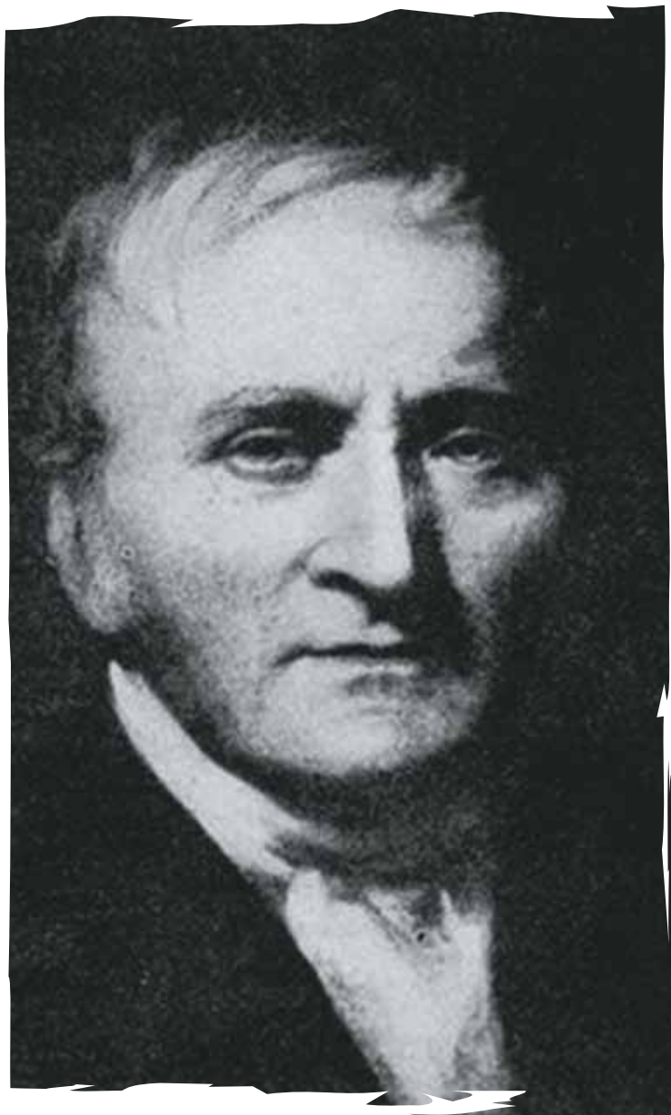
El modelo de la estructura atómica de Dalton se ha transformado a través del tiempo
